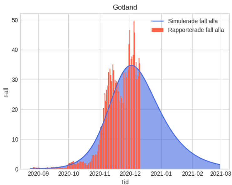
Figur 4. Gotlands län: Antal rapporterade och simulerade fall enligt scenario 0: 24 augusti 2020 – 1 mars 2021 (faktiskt rapporterade fall fram till 11 december).
